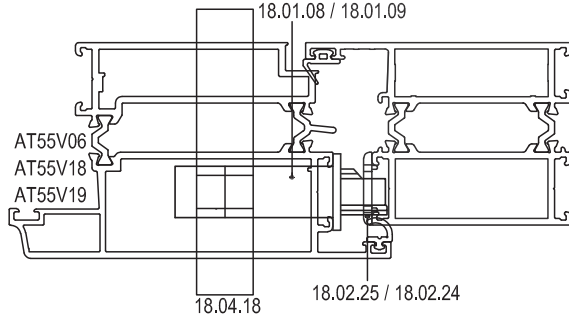
**DIŞA AÇILIM BİNİLİ ORTA BİRLEŞİM DETAYI İÇİN **OUTWARD OPENING FLUSH DOOR ADAPTER DETAIL
