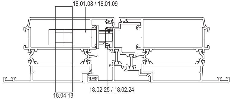
**İÇE AÇILIM BİNİLİ ORTA BİRLEŞİM DETAYI İÇİN **INWARD OPENING DOOR DETAIL
