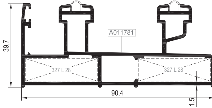
**RS83 F 03 Sineklik Kanadı için Kasa
