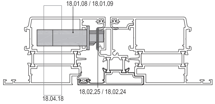
**İÇE AÇILIM BİNLİ ORTA BİRLEŞİM DETAYI İÇİN **INWARD OPENING DOOR DETAIL
